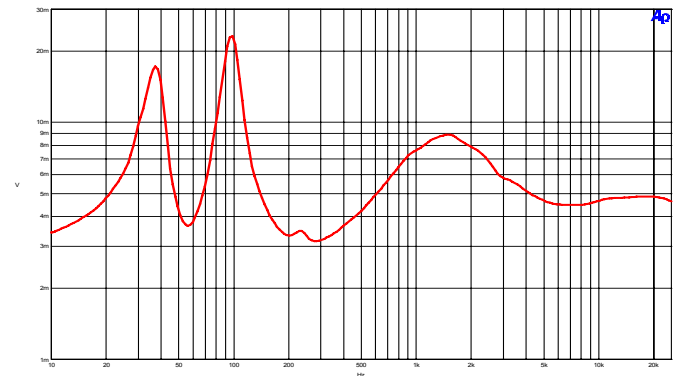
Impedanzkurve: Minimum 3,2 Ohm
