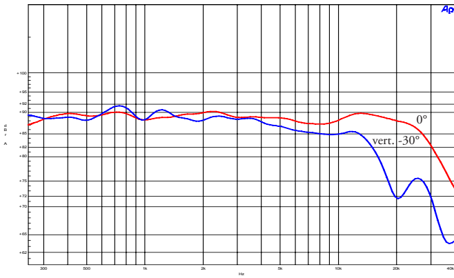
Frequenzgang: 30° aus der Achse, sehr gutes Abstrahlverhalten
