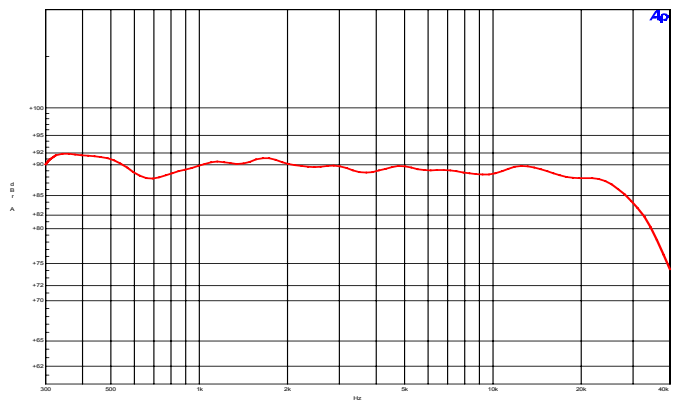
Frequenzgang: Mittel- Hochtonbereich
