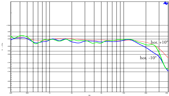
Frequenzgang: 10° hor. aus der Achse, fast keine Interferenzen
